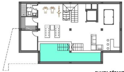
PLANTA SÓTANO
