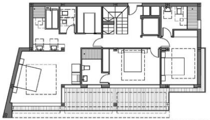
PLANTA PRIMERA
