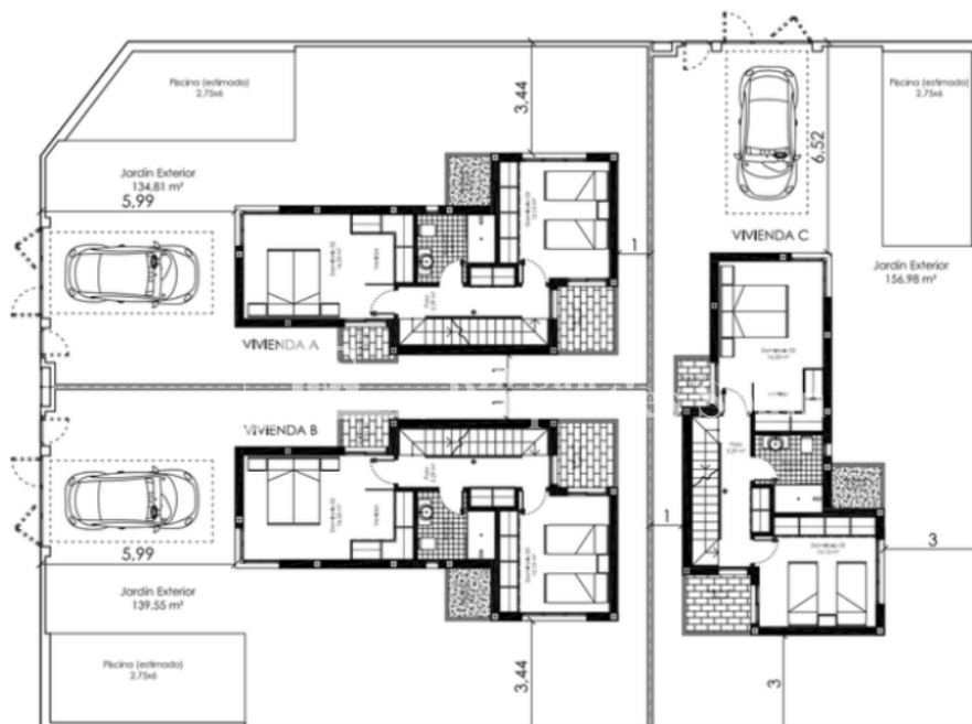
Planta Primera
