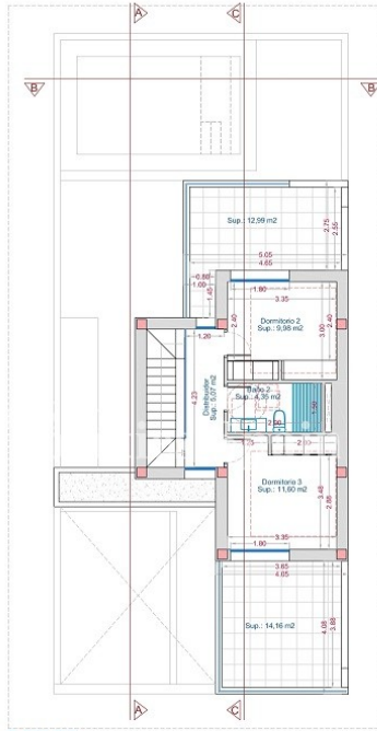
PLANTA PISO
