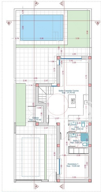
PLANTA BAJA
